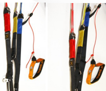
Unbeschleunigt - Beschleunigten
